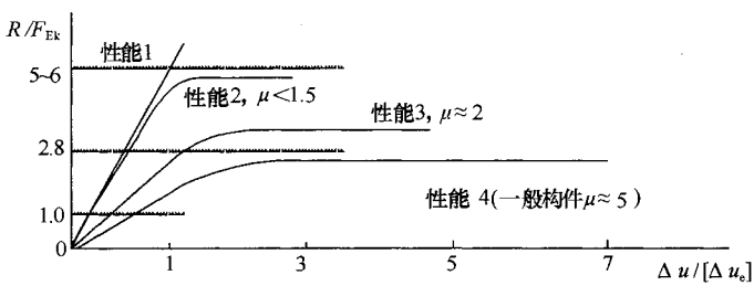
图 28 不同性能要求的位移和延性需求示意图
