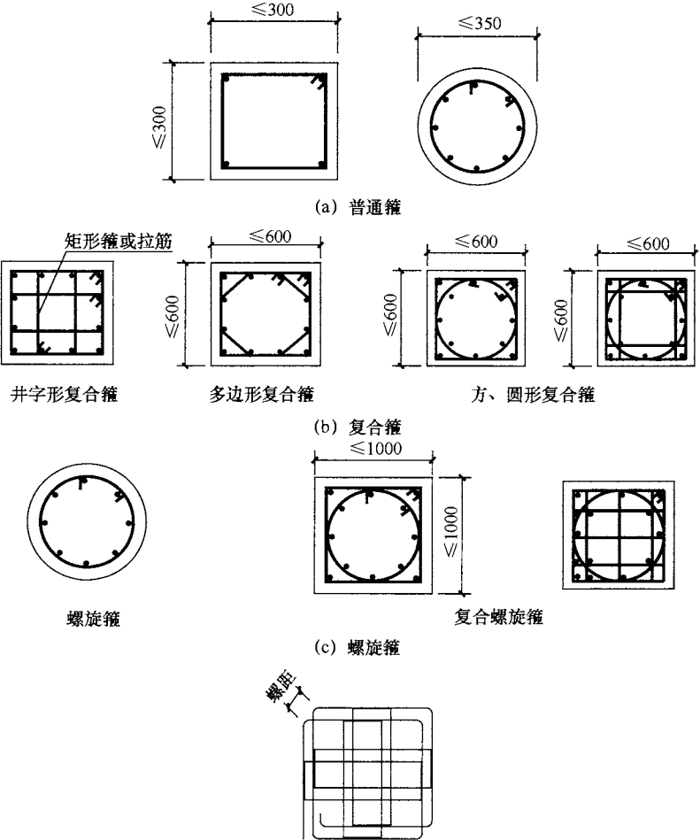
图 17 各类箍筋示意图
