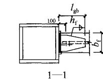
在上翼缘加楔形盖板, 板宽 = b_f - 3t_{gb}
