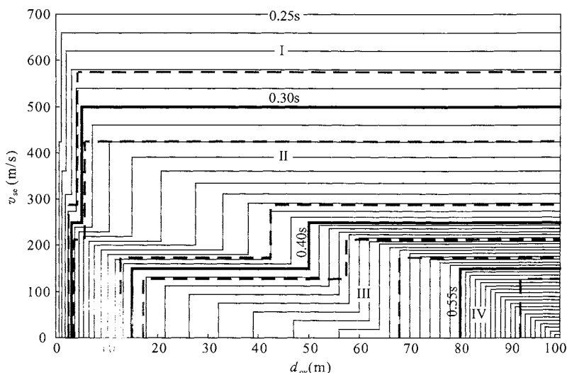
图 7 在 d_{ov} - v_{se} 平面上的 T_g 等值线图
