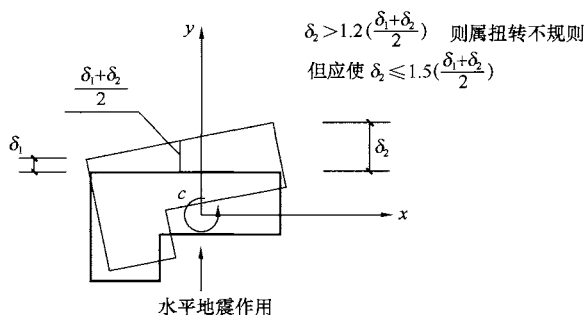
图 1 建筑结构平面的扭转不规则示例
